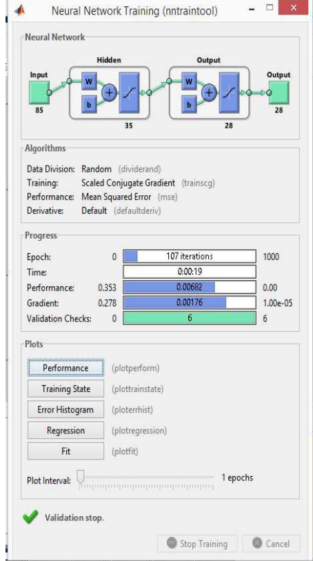
الشكل 8: (شبكات عصبونية الأداة)
